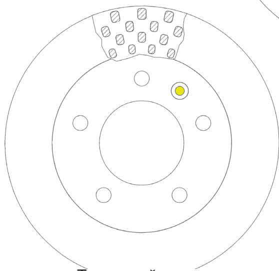
Тормозной диск с отверстием для малых стопорных винтов
