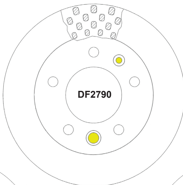
Тормозной диск с отверстиями для больших и малых стопорных винтов
