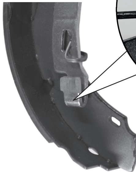
Конструкция TRW
