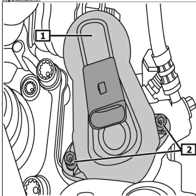
1 Nastawnik serwomotor
