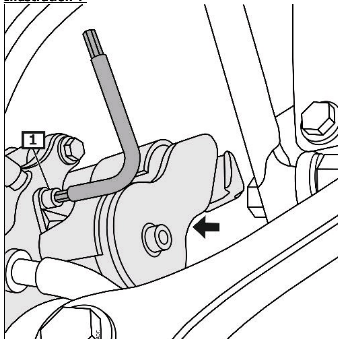
1 Vis (flèche)
