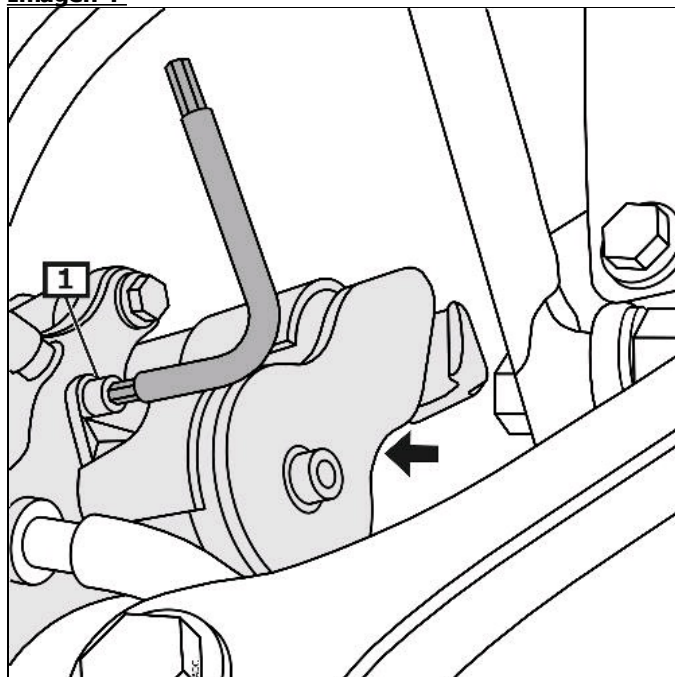
1 Tornillo(s) (flecha)
