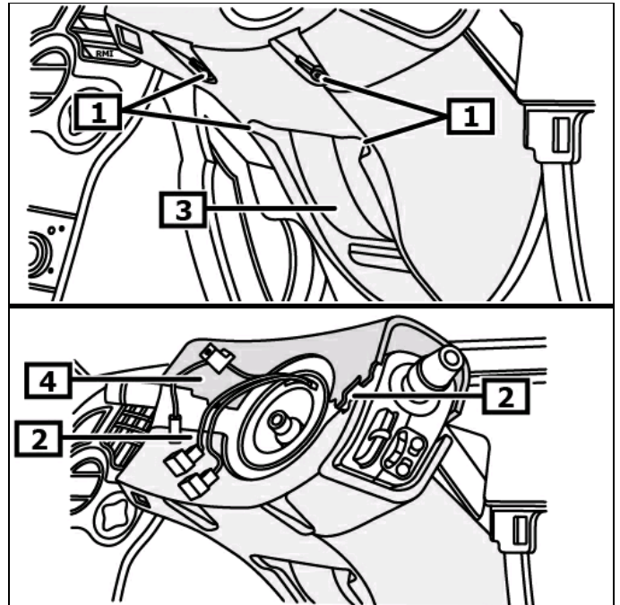
1 Kormányoszlop burkolat(ok) csavarja(i) alul
