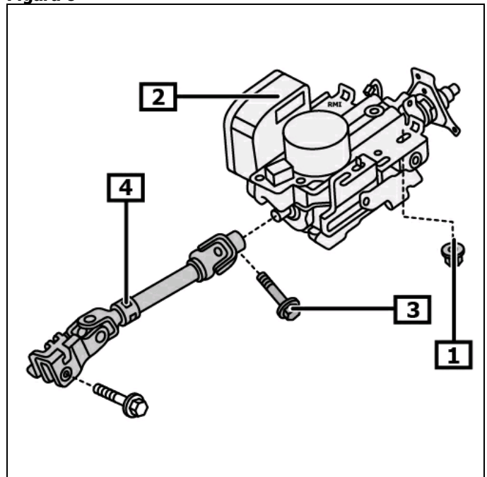
1 Piulița (piulițele) pentru coloana de direcție 2 Coloană de direcție
