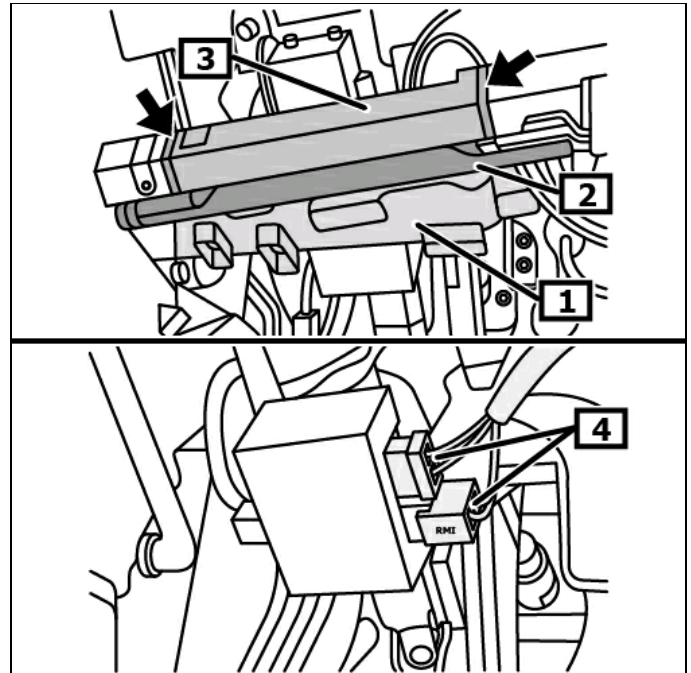
1 Conduit d'aération de l'espace pieds côté conducteur 2 Support pour le tableau de bord dans l'espace pieds 3 Support de la garniture de l'espace pieds 4 Connecteur(s) électrique(s)
