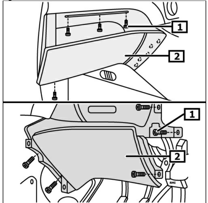
1 vite(i) copertura
