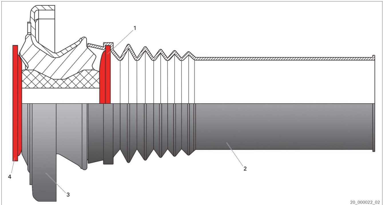
1. ábra: Toronycsapágy szervizkészttel
