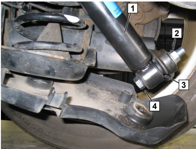
Slika 2: Vgrajen blažilnik udarcev
