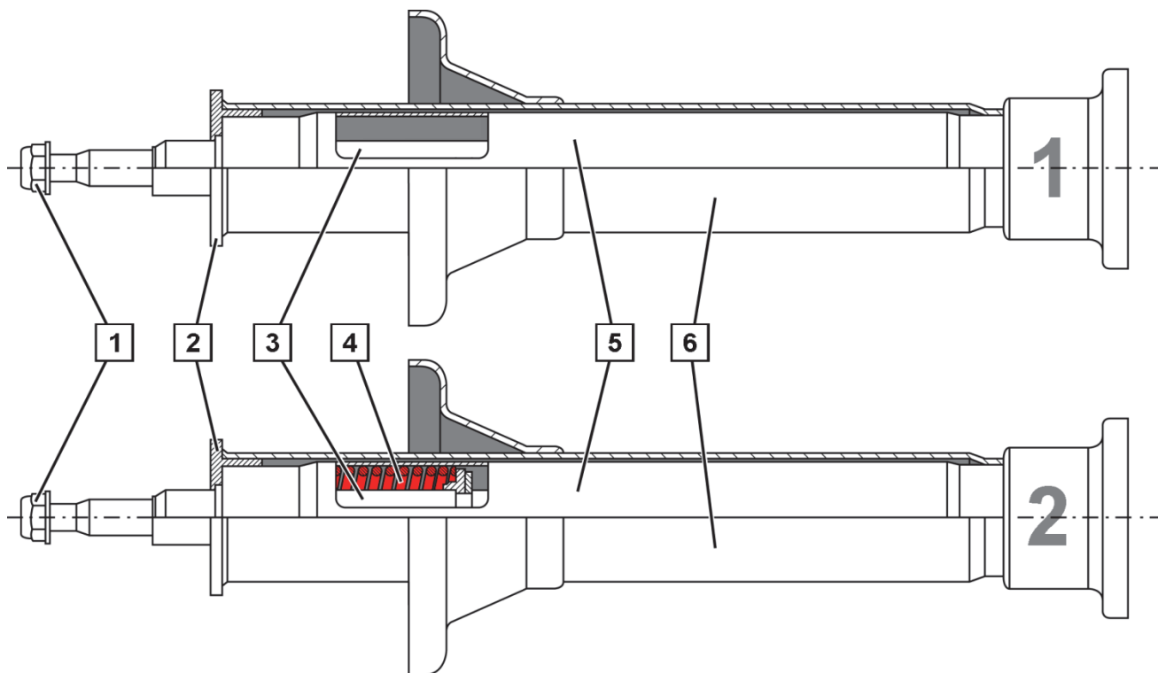
Sl. 1: Amortizer 1 bez odbojne opruge | Amortizer 2 sa odbojnom oprugom
