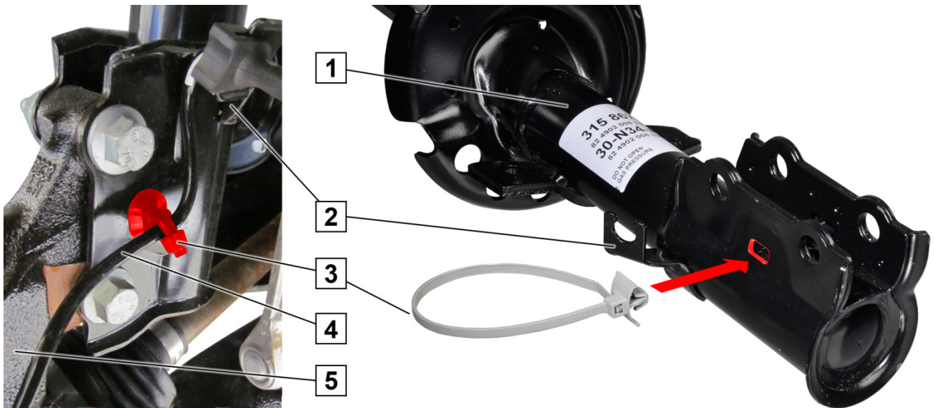
Fig. 1: Fixarea cablului ABS cu colier pentru cabluri (3)
