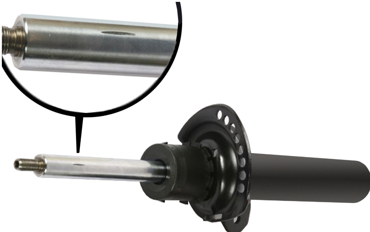
Fig. 1: Tige de piston avec rainure de pressurisation
