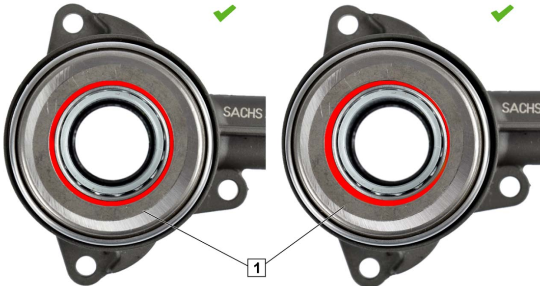
Obr. 2: CSC so samocentrováním. Ložisko centované a necentované (príklad).
