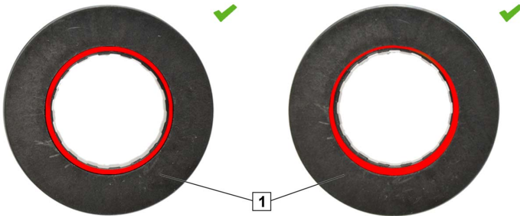
Sl. 1: Sistem za odvajanje kvačila sa samocentriranjem. Ležaj centriran i necentriran (primer).
