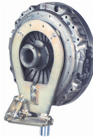
obr. 3: Montážní pomůcka pro přítlačný kotouč Blitz Rotary čís. mat. 101758
