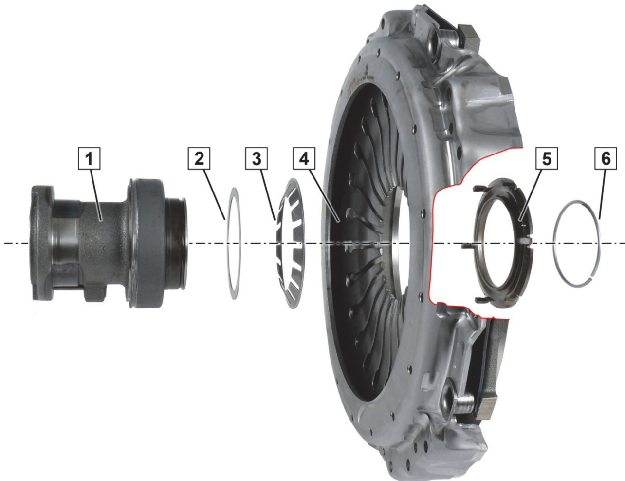
Sl. 1: Potisni ležaj s fiksnim spojem. Vrstni red montaže in naravnost delov.
