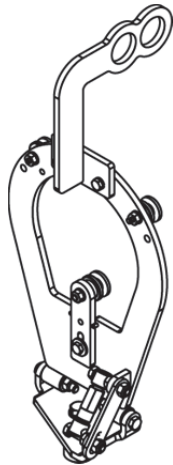
Bild 1: Monteringshjälpmedel med transportbygel cDISK Blitz Rotary art.nr. 3745410
