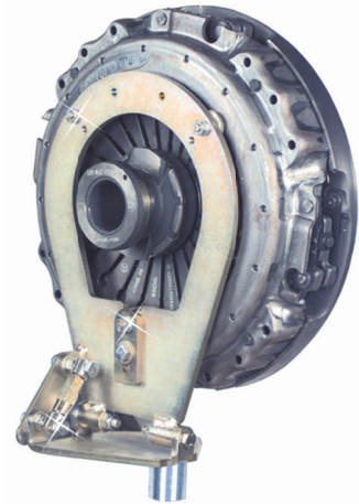
Fig. 3: Monteringshjelp trykkplate Blitz Rotary art.nr. 101758
