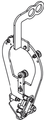
Fig. 1: Monteringshjelp med transporthåndtak cDISK Blitz Rotary art.nr. 3745410
