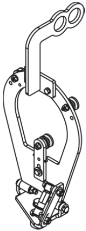
Sl. 1: Pomagalo pri montaži s drškom za transport cDISK Blitz Rotary br. art. 3745410
