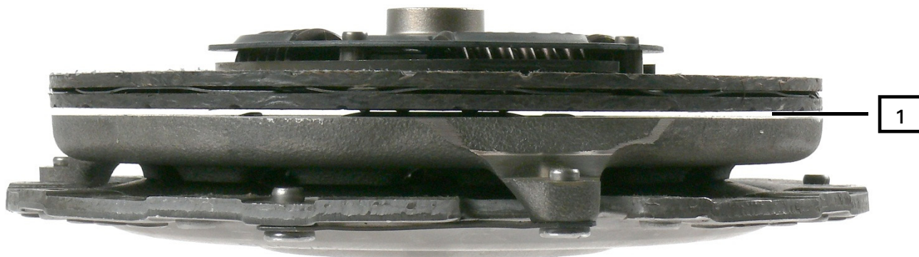
1. ábra: MX tengelykapcsoló
