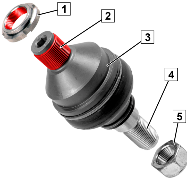
Εικ. 1: Άρθρωση ανάρτησης
