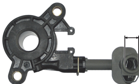
SI. 2: CSC 3182 600 129 → 3182 654 146 prečnik hidrauličkog priključka 13,3 mm
