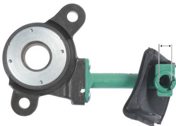
SI. 3: CSC 3182 600 120 prečnik hidrauličkog priključka 12,2 mm
