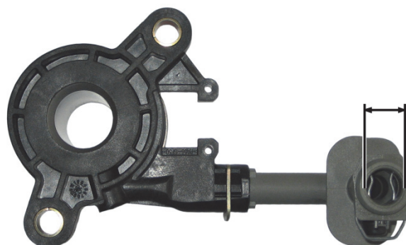
Рис. 2: CSC 3182 600 129 → 3182 654 146 Диаметр штуцера гидросистемы 13,3 мм
