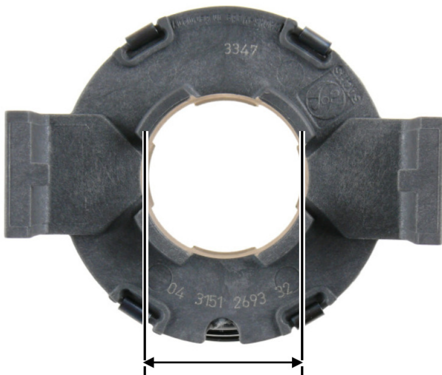
Ilustracja 1: Wyprzęgnik
