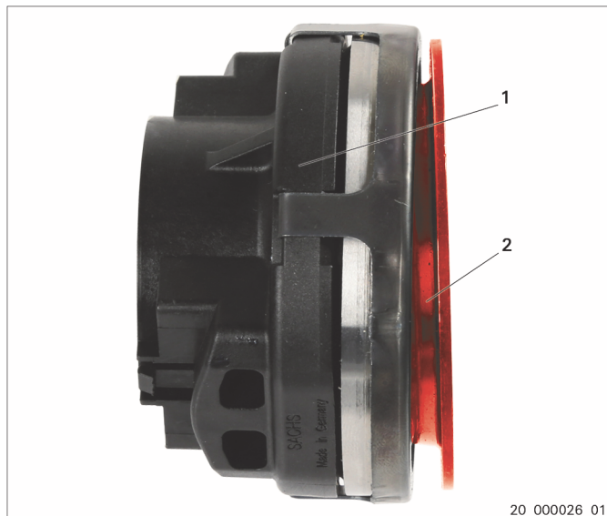
1. att.: izspiedējs ar brīvkustības izlīdzināšanas mehānismu
