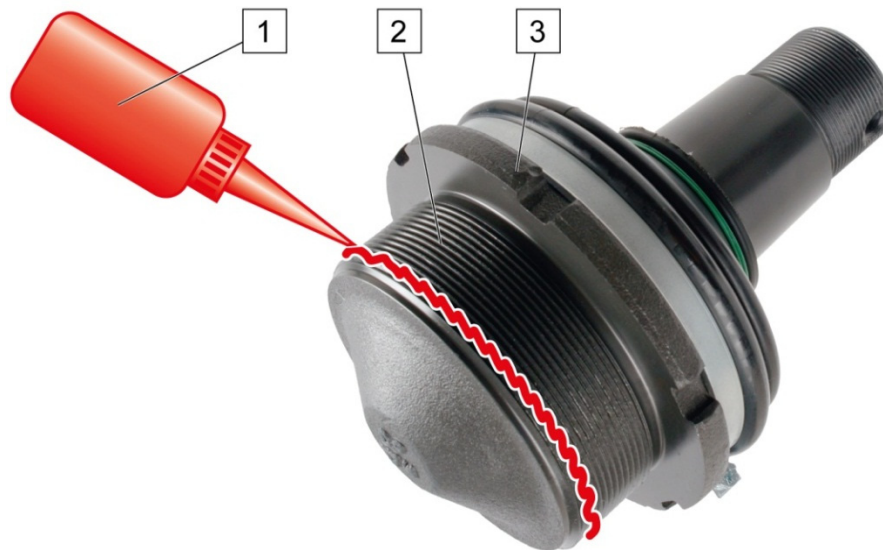
Rys. 1: Przegub nośny, środek do zabezpieczania gwintów
