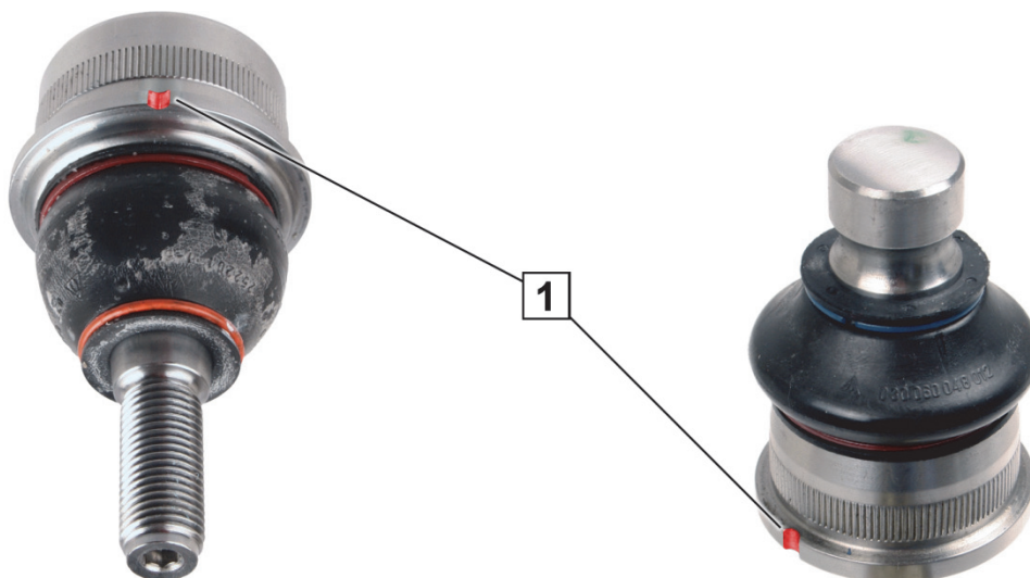
Rys. 1: Przegub nośny z karbem (wahacz poprzeczny u góry)
