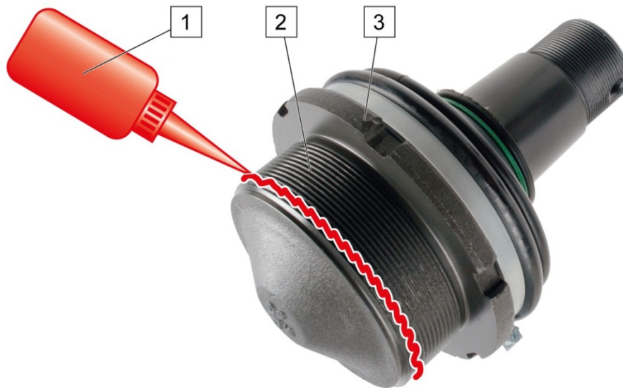
Fig. 1: Bærehengsel, middel for sikring av gjenger
