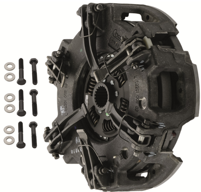
Fig. 2: Embreagem, construção alterada
