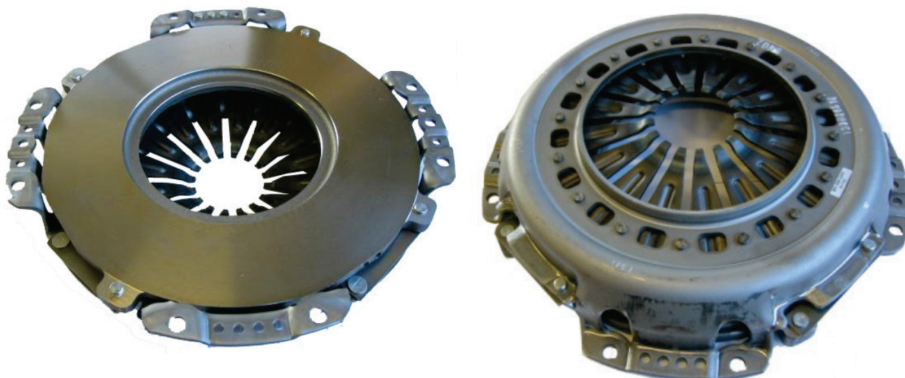
Fig. 1: 330 mm enkelt-membrankobling
