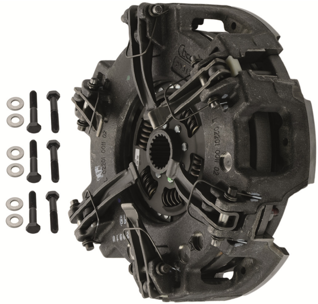
图 2：离合器，结构改进
