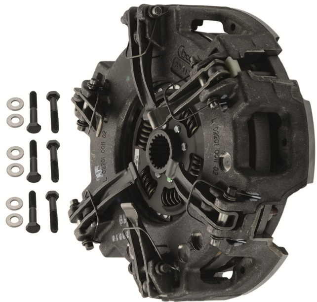
Фиг. 2: Съединител, променена конструкция
