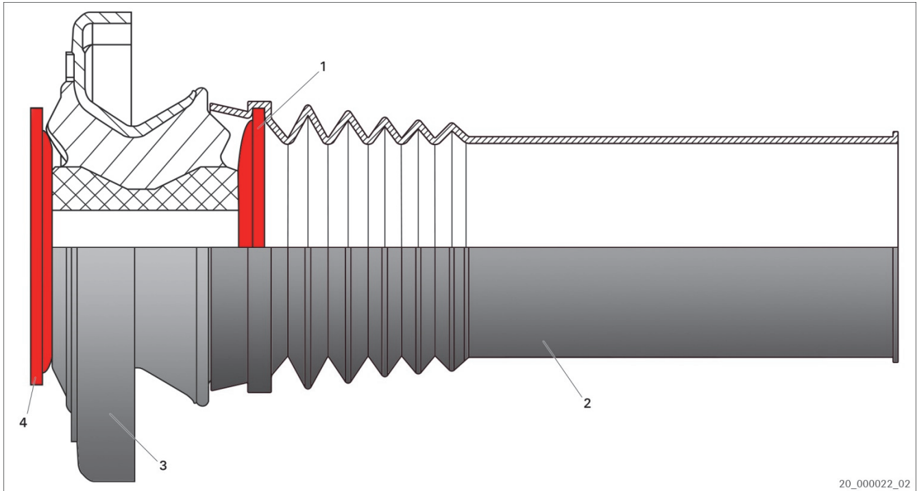
Sl. 1: Potporni ležaj opružne noge sa servisnim kompletom
