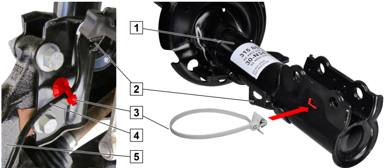
1. ábra: ABS-kábel rögzítése kábelkötővel (3)
