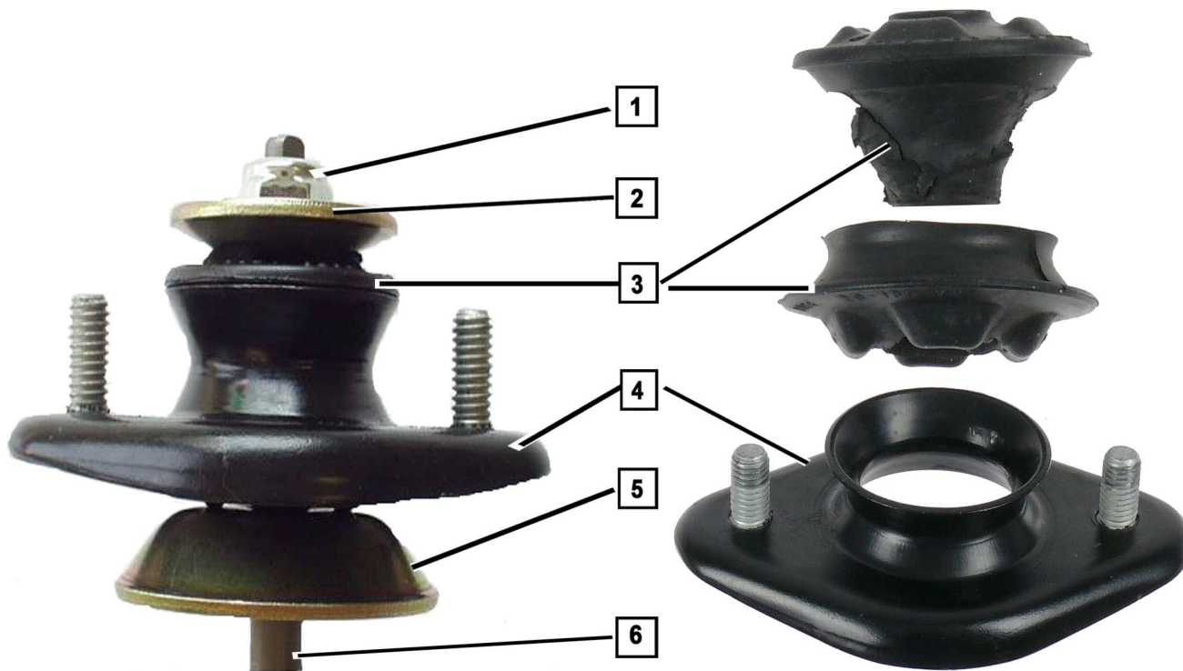
1. ábra: Sértetlen toronycsapágó kapcsolódó alkatrészekkel
