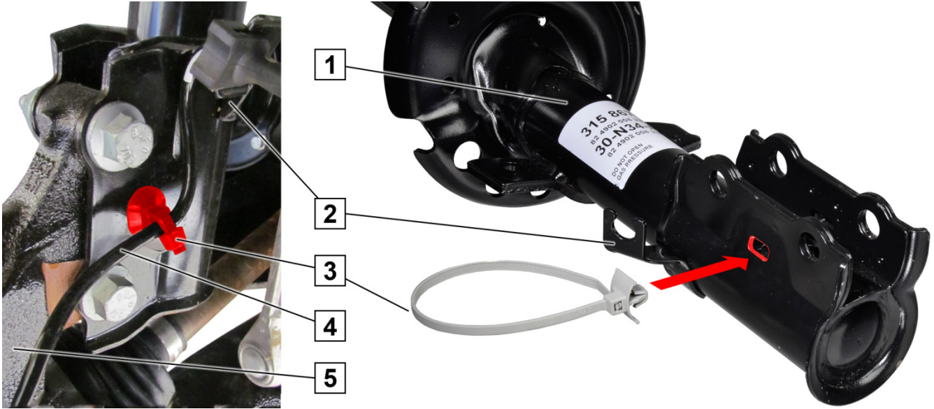
Şek. 1: ABS kablosunu kablo bağı (3) ile sabitleyin
