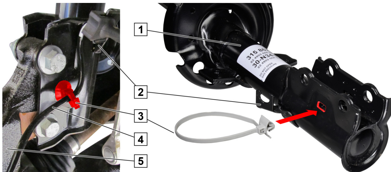
Obr. 1: Kabel ABS upevnit pomocí stahovací kabelové pásky (3)
