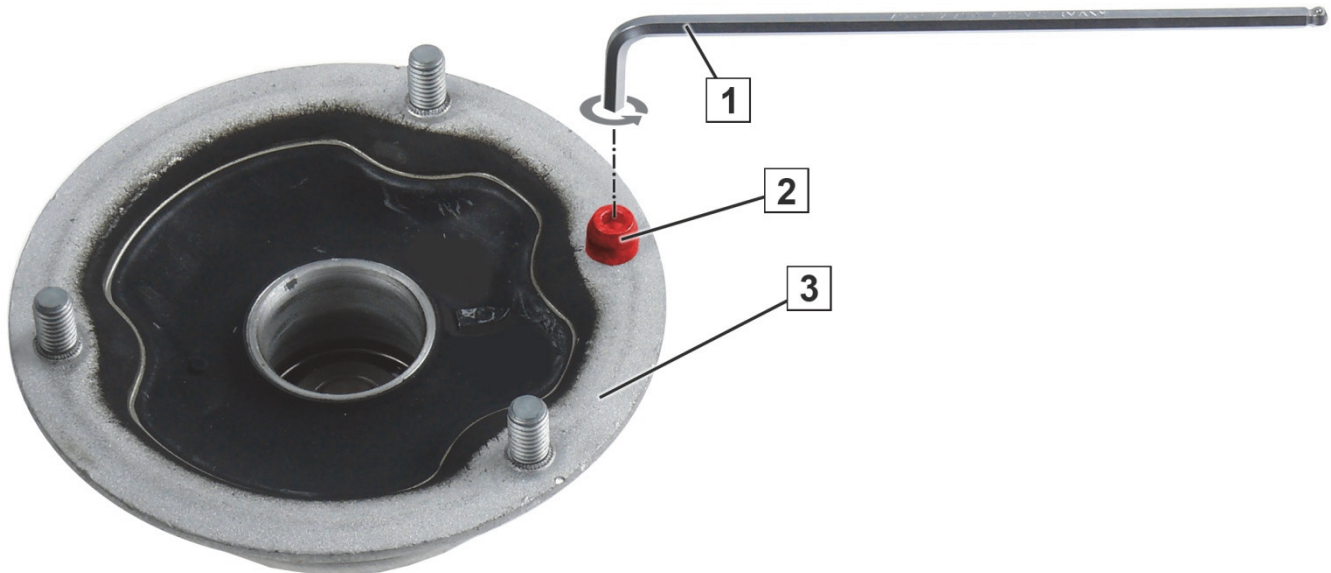
Sl. 1: Ležaj za oslanjanje sa pinom za pozicioniranje
