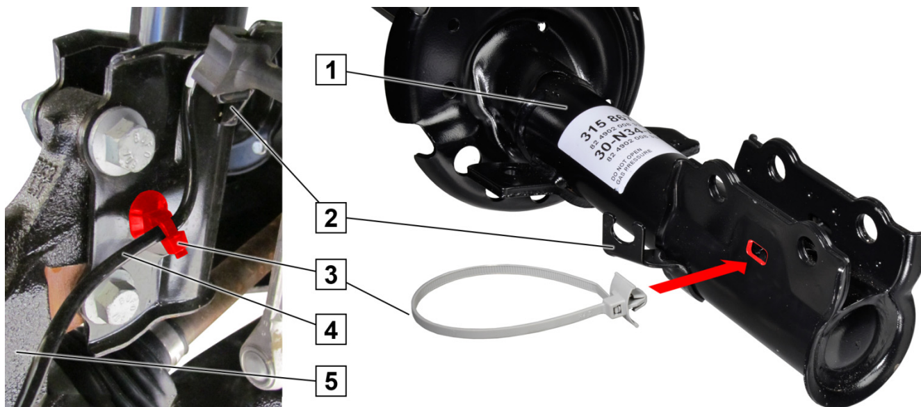
Rys. 1: Montaż przewodu ABS za pomocą opaski kablowej (3)
