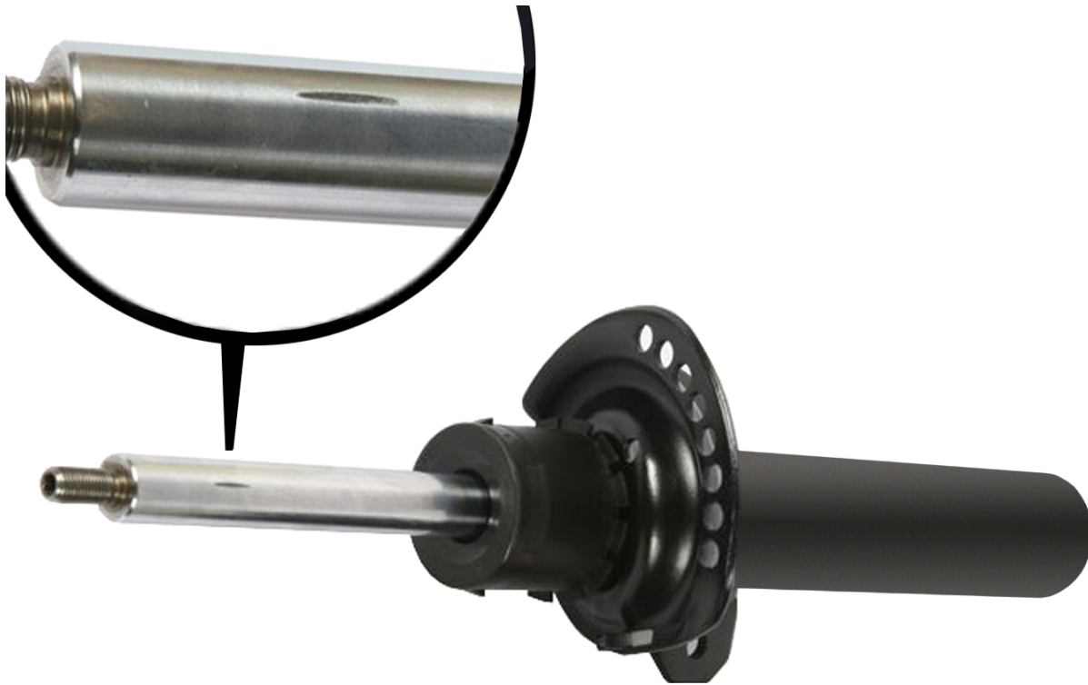
Afb. 1: Zuigerstang met groef
