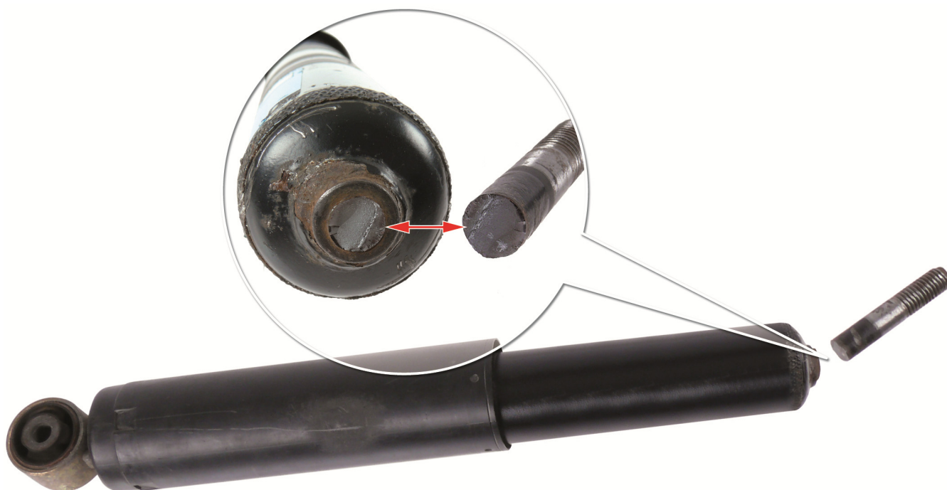
Sl. 1: Prijelom vijka zgloba uslijed promjenjivog opterećenja savijanjem
