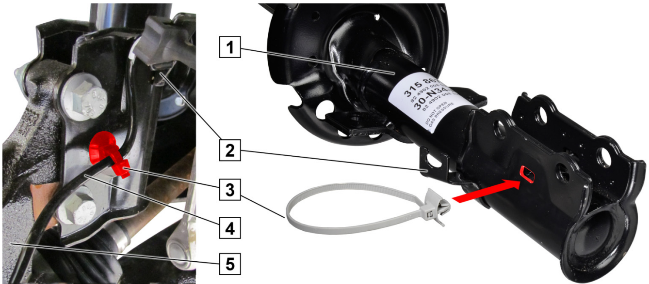
Sl. 1: Učvršćivanje ABS kabela kablskom vezicom (3)
