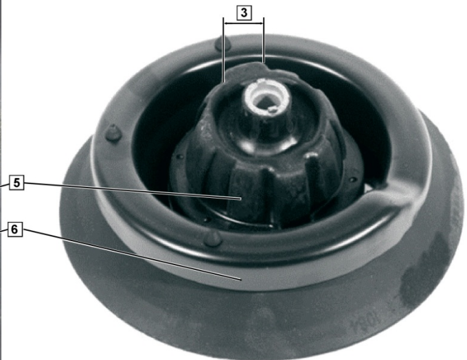
Εικ. 3: Έδρανο γόνατου ανάρτησης
