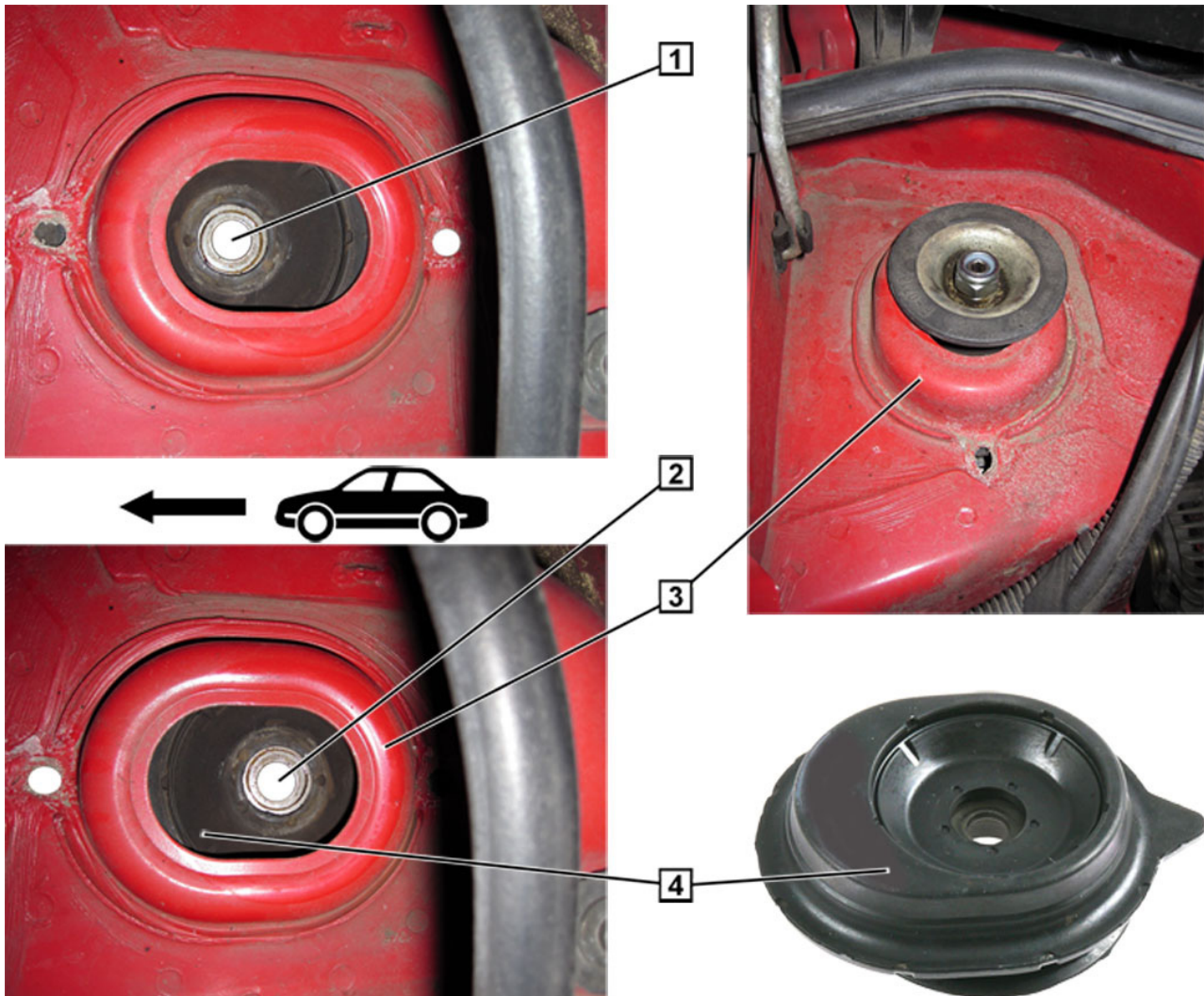
Fig. 1 : Support de jambe de force dans de différentes positions de montage
