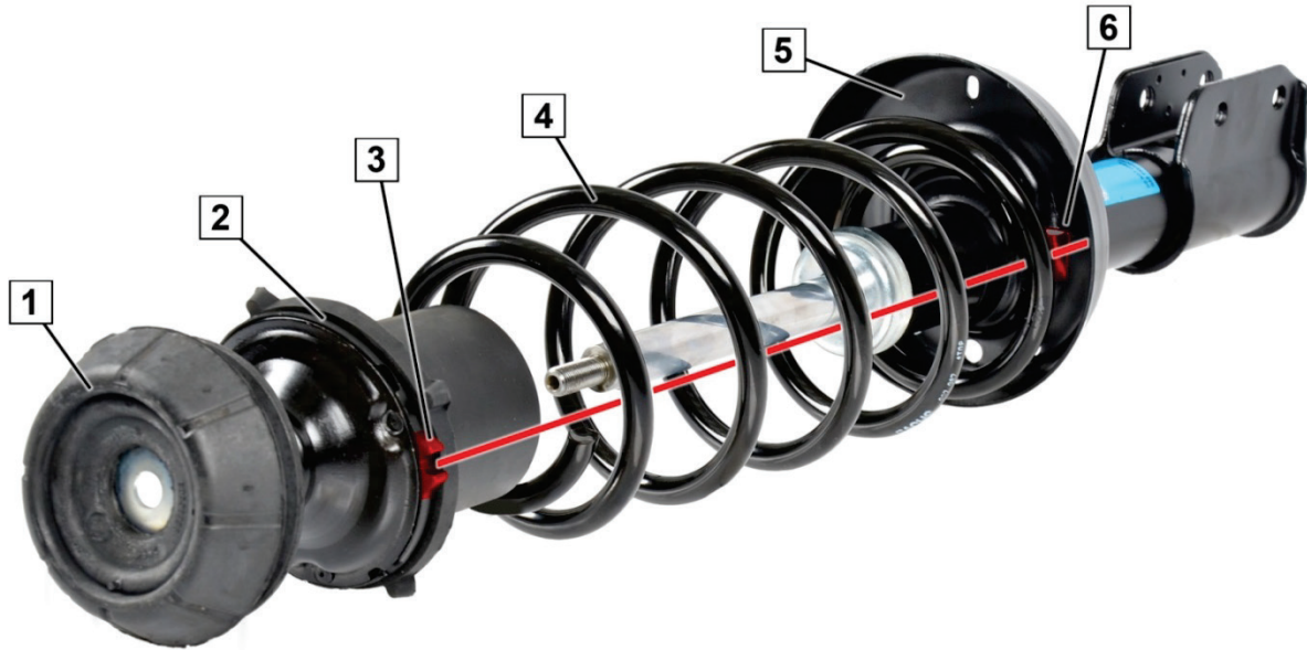
Kuva 1: Joustintuen tukilaakeri oikein asennettuna
