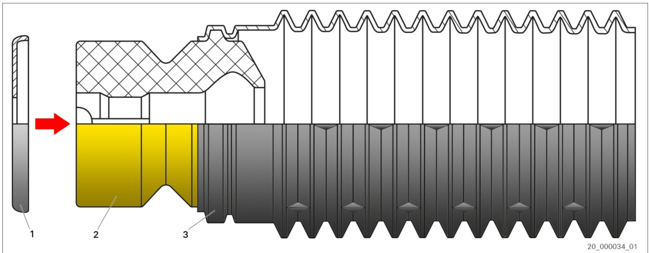
Abb. 1: Service-Kit mit Metallkappe
