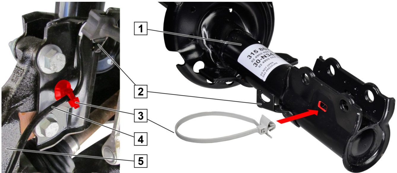
Fig. 1: Fastgør ABS-kablet med kabelbinder (3)
