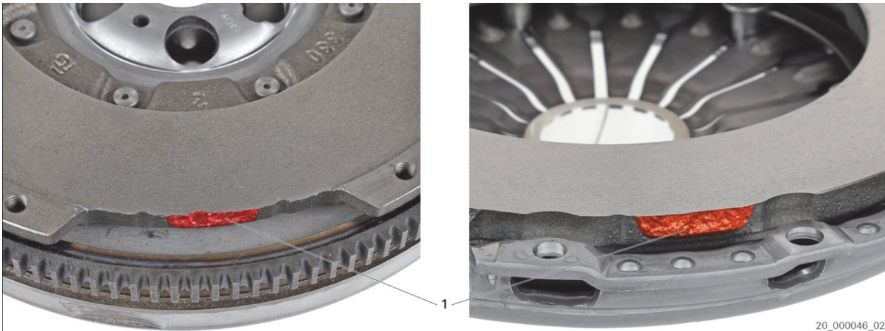
1. ábra: Törési él (példa)
